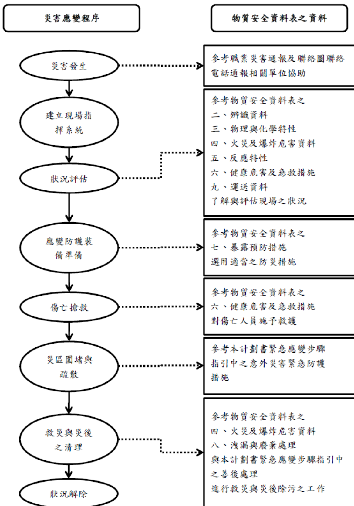
附表 1 化學災應變程序與安全資料表(原稱物質安全資料表)之對照應用(參考例)
